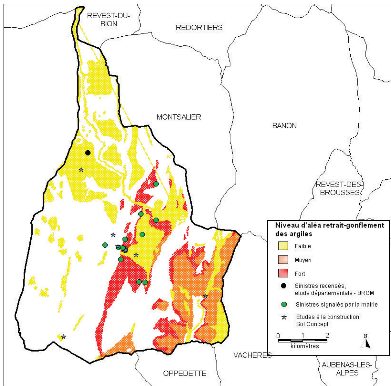
Illustration 7 : Carte d'aléa retrait-gonflement des argiles sur la commune de Simiane-la-Rotonde
